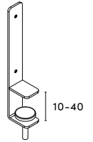
Okucie / Fitting 28x40x200
