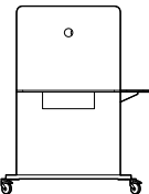
120 x 40 H.180 cm 47¼" x 15¾" H.70¾" Mod. FLIPPER su ruote Flipper on castors - Flipper sur roulettes - Flipper auf Rollen - Flipper op wielen - Flipper sobre ruedas 48 x 28 H.1,8 cm 18¾" x 11" H.¾" Mensola Flipper Flipper shelf - Étagère pour Flipper - Konsole für Flipper - Plank voor Flipper - Estante para Flipper
