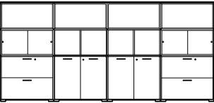
320 x 40 H.151 cm 126" x 15¾" H.59½" Contentitori mod. UBI EVO UBI EVO Containers - Cubes UBI EVO - Container UBI EVO - Containers UBI EVO - Contenedores UBI EVO
