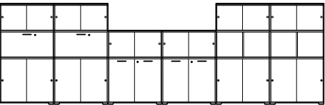
482 x 40 H.151 cm 189¾" x 15¾" H.59½" Contentitori mod. UBI EVO UBI EVO Containers - Cubes UBI EVO - Container UBI EVO - Containers UBI EVO - Contenedores UBI EVO
