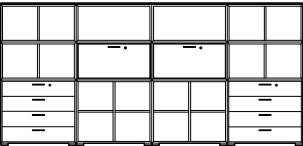
320x40 H.151 cm 126" x 15¾" H.59½" Contentitori mod. UBI EVO UBI EVO Containers - Cubes UBI EVO - Container UBI EVO - Containers UBI EVO - Contenedores UBI EVO
