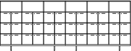
482 x 40 H.184 cm 189¾" x 15¾" H.72½" Contentitori mod. UBI EVO UBI EVO Containers - Cubes UBI EVO - Container UBI EVO - Containers UBI EVO - Contenedores UBI EVO
